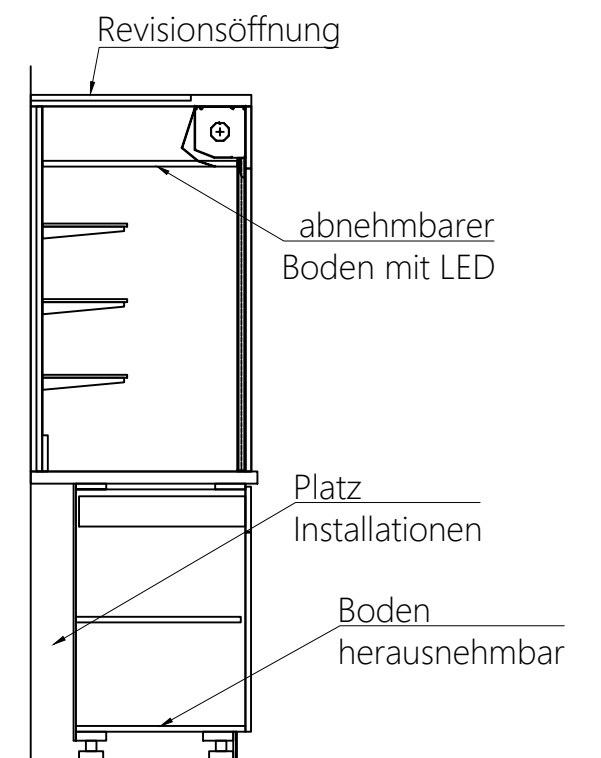
Schnitt Rückbereich Theke
