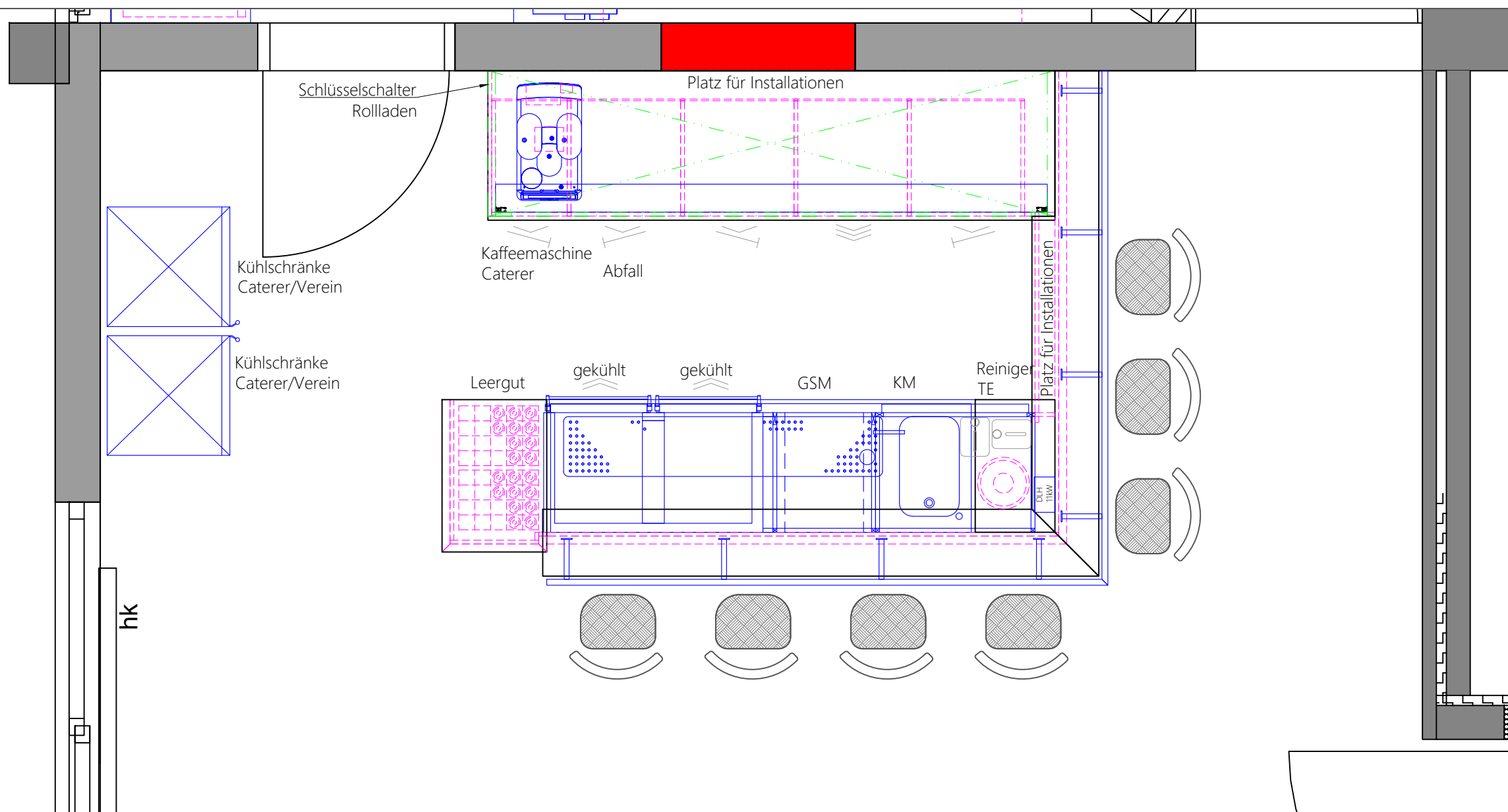
Thekenansicht ohne Rückbereich
